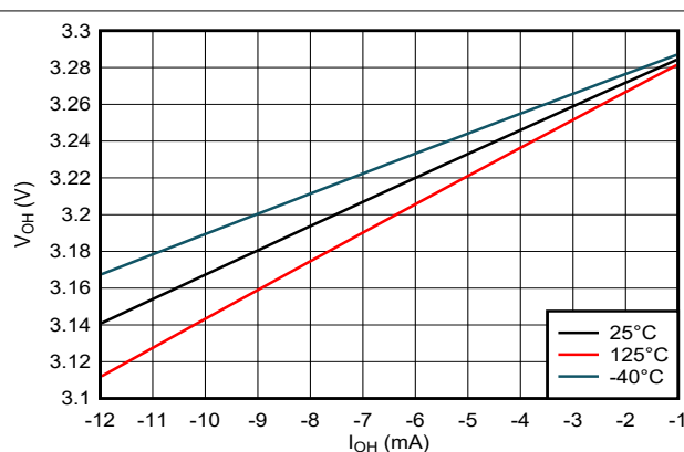
图 5-8. 高电平状态下输出电压与电流间的关系 (3.3V 电源)
