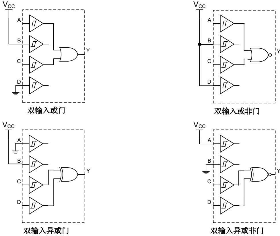
图 7-2. 逻辑配置
