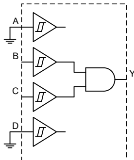
双输入与门
