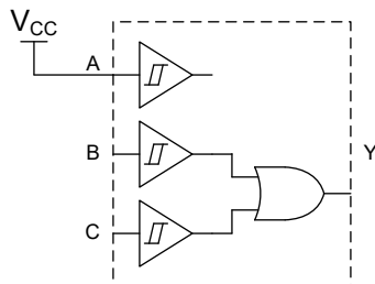
双输入或门
