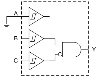
具有 1 个反相输入的双输入与门
