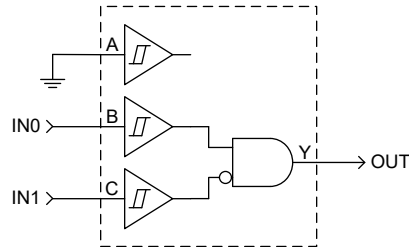
图 8-1. 典型应用原理图
