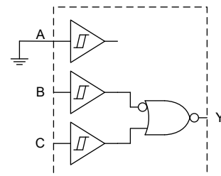
具有 1 个反相输入的双输入或非门
