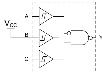
具有 1 个反相输入的双输入与非门
