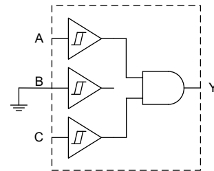
双输入与门
