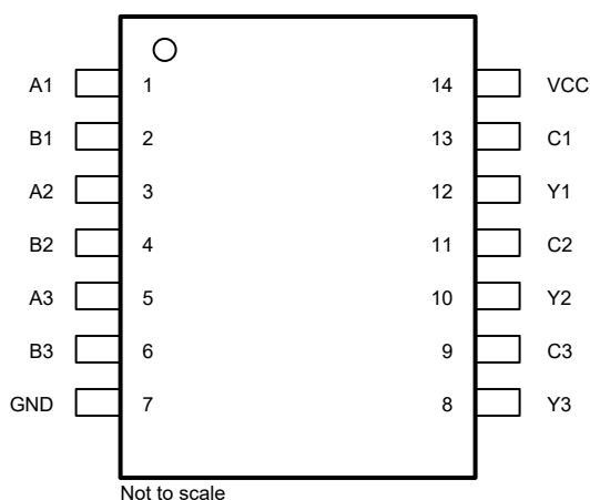
图 4-1. SN74AC3G98 PW 封装，14 引脚 TSSOP ( 顶视图 ) 图 4-2. SN74AC3G98 BQA 封装，14 引脚 WQFN ( 顶视图 )
