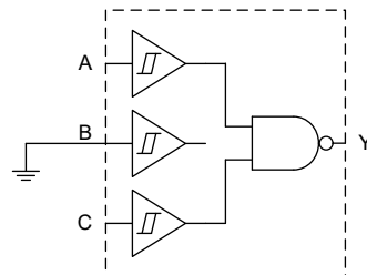
双输入与非门
