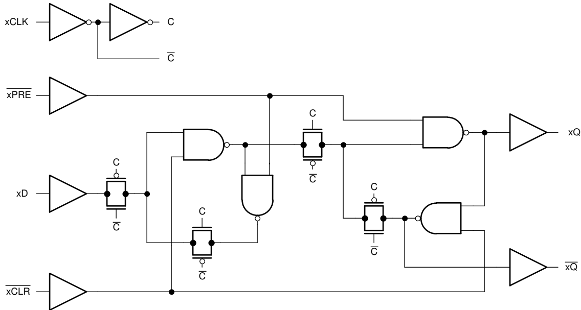
图 7-1. SN74AC74-Q1 的一个通道的逻辑图 (正逻辑)
