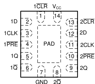
BQA 封装， 14 引脚 WQFN (透明顶视图)
