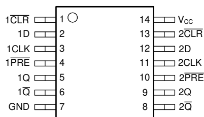
PW 封装， 14 引脚 TSSOP (顶视图)
