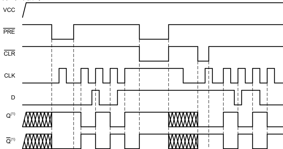
时序图
