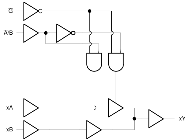
逻辑图
