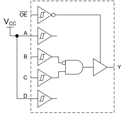
具有 1 个反相输入的双输入与门
