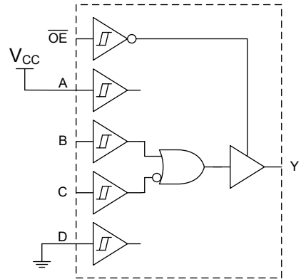
具有 1 个反相输入的双输入或门
