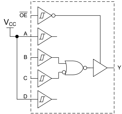
具有 1 个反相输入的双输入或非门
