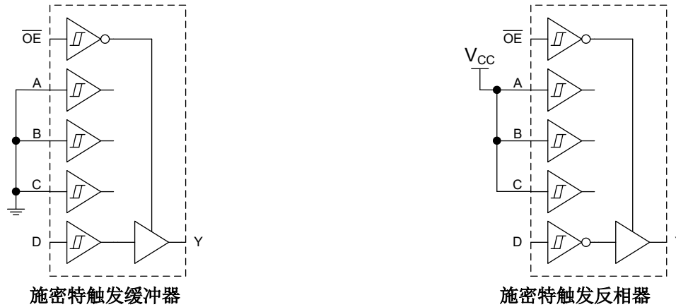
图 7-1. 逻辑配置
