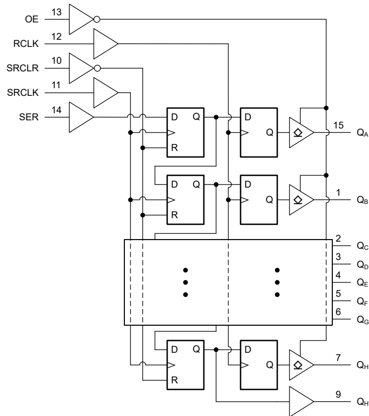
图 7-1. SN74ACT596 的逻辑图 (正逻辑)
