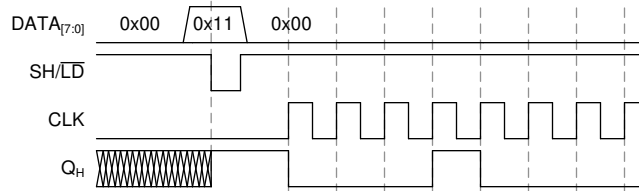
图 8-2. 应用时序图
