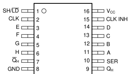
图 4-1. PW 封装， 16 引脚 TSSOP (顶视图)
