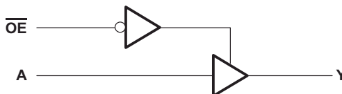
简化逻辑图 (正逻辑)
