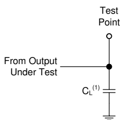
图 7-1. 推挽输出的负载电路
