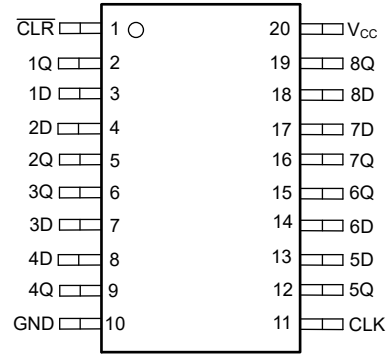
图 4-2. SN74AHC273-Q1 PW、DGS 封装 (顶视图)
