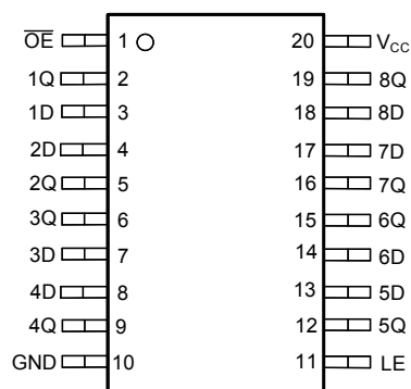
图 4-2. SN74AHC373-Q1 PW、DGS 封装 (顶视图)
