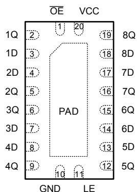
图 4-1. SN74AHC373-Q1 RKS 封装 (顶视图)
