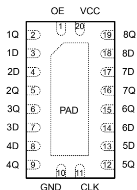
图 4-1. SN74AHC374-Q1 RKS 封装 (顶视图)
