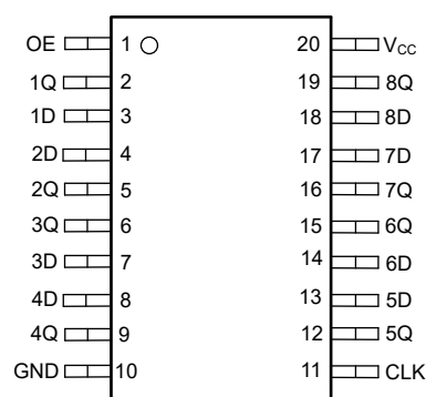
图 4-2. SN74AHC374-Q1 PW、DGS 封装 (顶视图)
