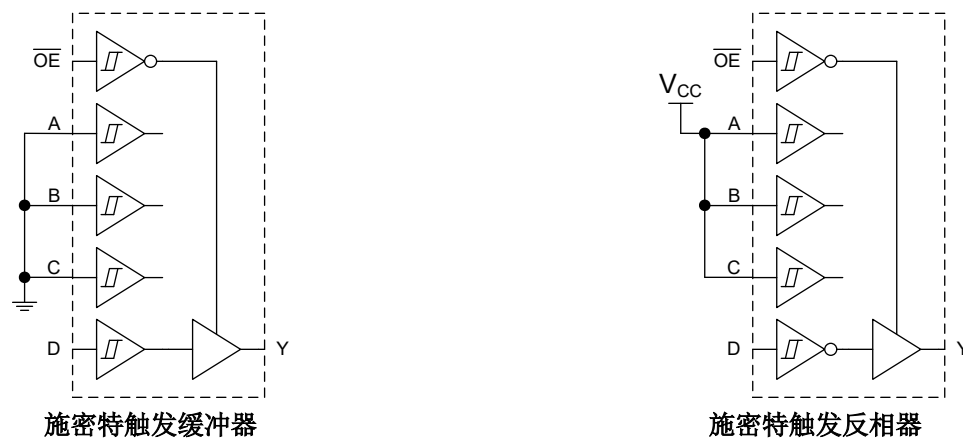
图 7-1. 逻辑配置
