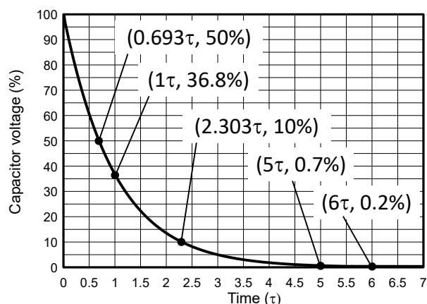
图 8-2. 应用时序图
