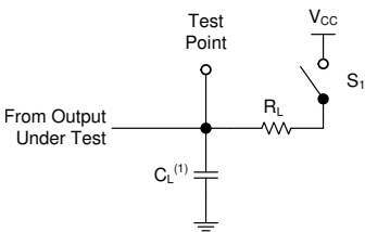
图 6-1. 开漏输出的负载电路
