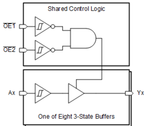
功能方框图
