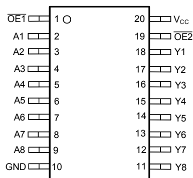
图 4-2. SN74AHC9541-Q1 PW、DGS 封装 (顶视图)
