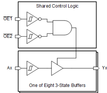
图 7-1. 施密特触发器输入图
