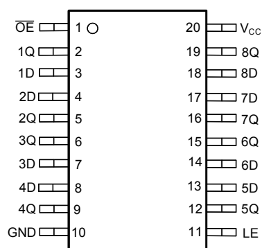
图 4-2. SN74AHCT373-Q1 PW、DGS 封装 (顶视图)
