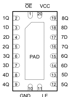
图 4-1. SN74AHCT373-Q1 RKS 封装 (顶视图)
