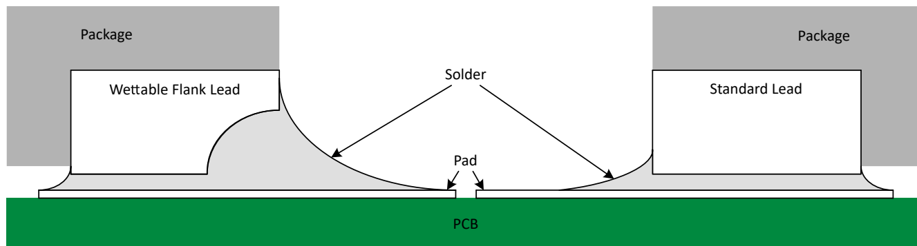
图 6-1. 焊接后具有可润湿侧翼的 QFN 封装和标准 QFN 封装的简化剖面图
