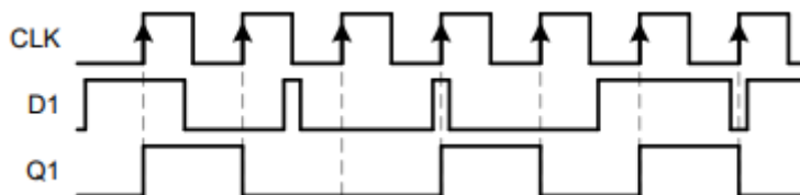
图 7-2. 显示时钟运行的简化功能图
