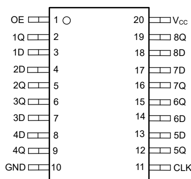
图 4-2. SN74AHCT374-Q1 PW、DGS 封装 (顶视图)
