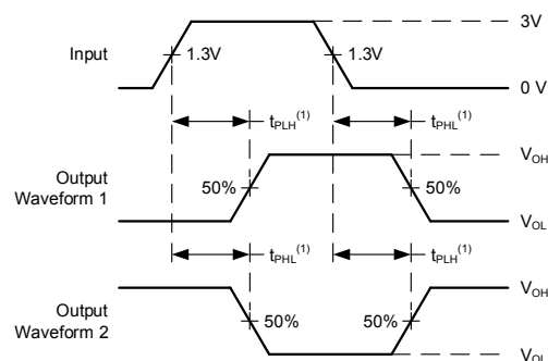
图 6-2. 电压波形传播延迟
