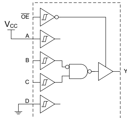
具有 1 个反相输入的双输入与非门
