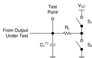
图 6-1. 三态输出的负载电路
