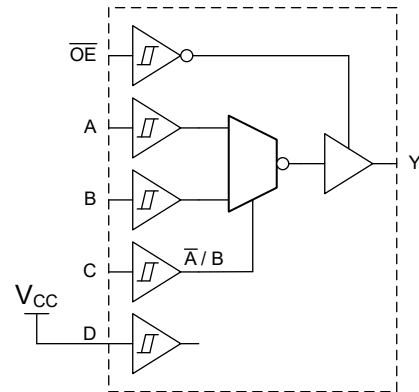
具有反相输出的 2:1 数据选择器
