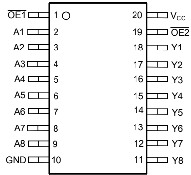
图 4-2. SN74AHCT540-Q1 PW、DGS 封装 (顶视图)
