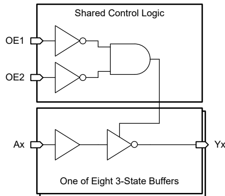
功能方框图
