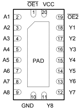
图 4-1. SN74AHCT540-Q1 RKS 封装 (顶视图)
