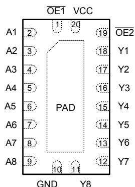
图 4-1. SN74AHCT7541-Q1 RKS 封装 (顶视图)
