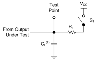
图 6-1. 开漏输出的负载电路
