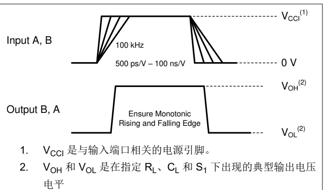
图 6-3. 输入转换上升或下降速率
