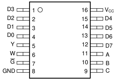
D 或 PW 封装 16 引脚 SOIC 或 TSSOP 顶视图
