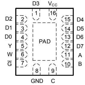
WBQB 封装 16 引脚 WQFN 俯视图
