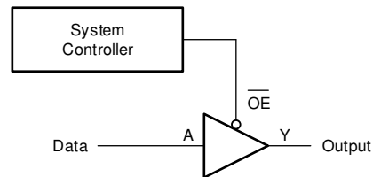
图 8-1. 典型应用框图
