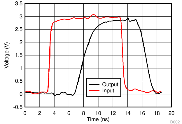
图 5-2. 50MHz 下的开关特性 出色的信号完整性
