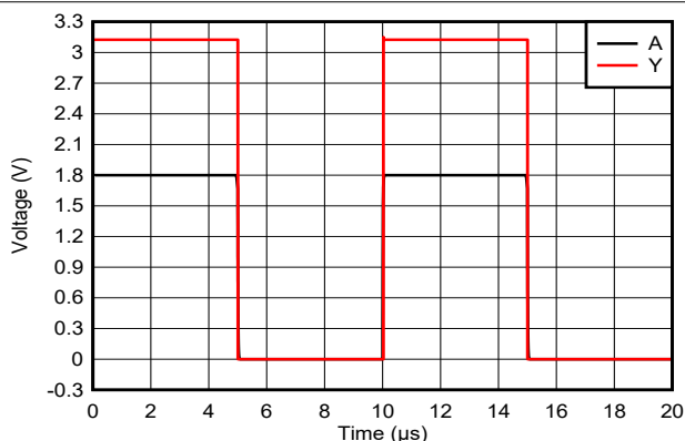
图 8-2. 应用时序图
