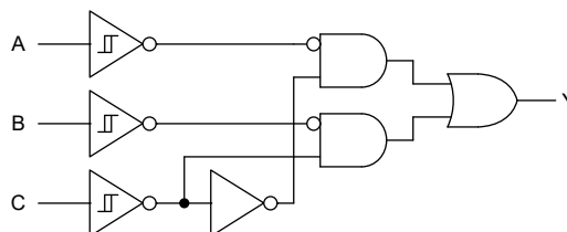
简化逻辑图
