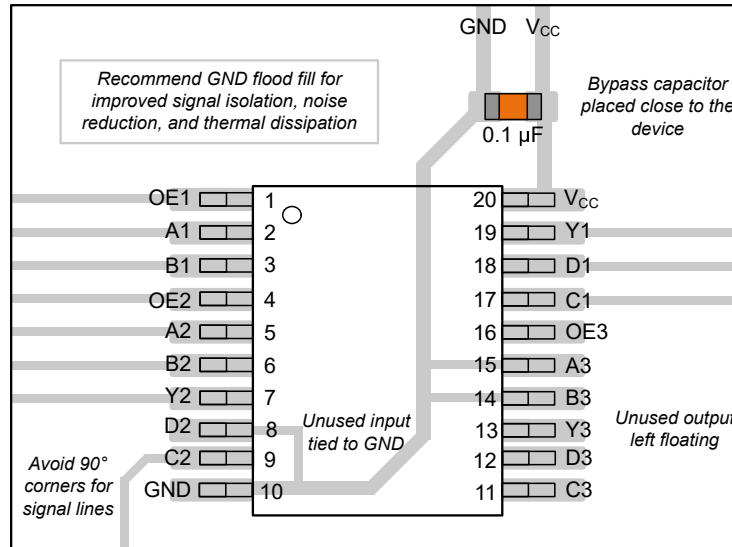
图 10-3. SN74LV3T99-Q1 采用 TSSOP 封装的示例布局
