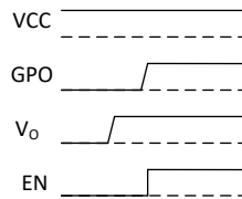
图 10-2. 典型应用时序图
