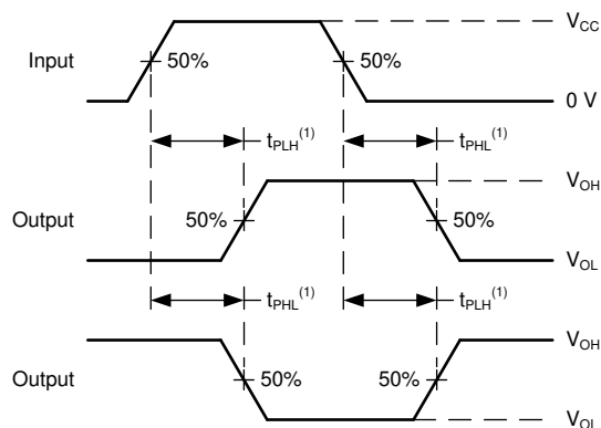
图 7-4. 电压波形传播延迟
