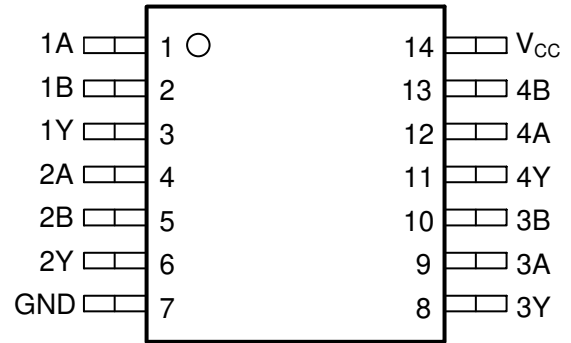
图 5-2. PW 封装，14 引脚 TSSOP (顶视图)
