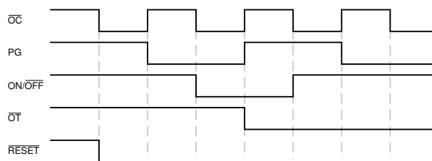
图 10-2. 应用时序图
