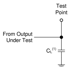
图 7-1. 推挽输出的负载电路
