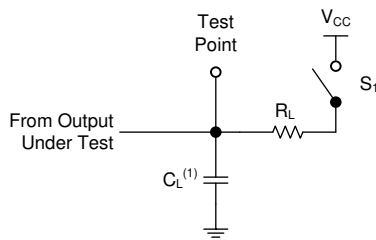
图 7-1. 开漏输出的负载电路
