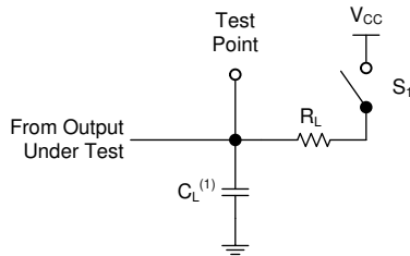
图 7-1. 开漏输出的负载电路
