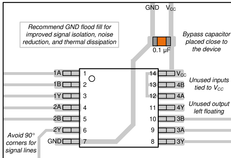
图 11-1. SN74LV6T17 的示例布局
