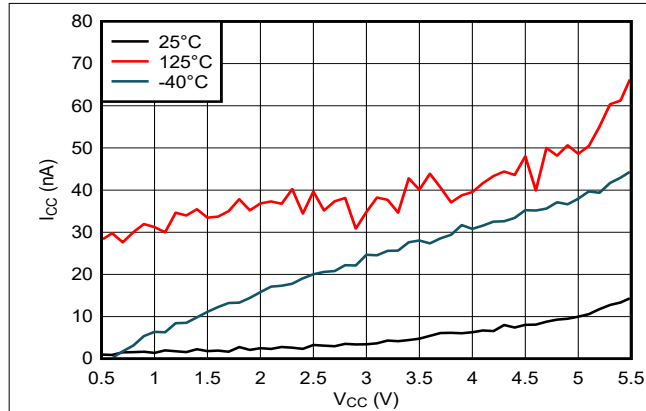
图 7-3. 电源电压两端的电源电流
