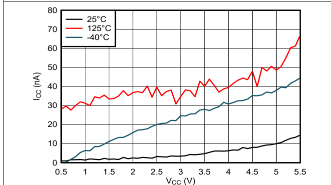
图 5-3. 电源电压两端的电源电流
