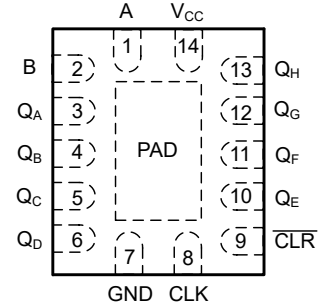
图 4-2. BQA 封装，14 引脚 WQFN ( 透明顶视图 )
