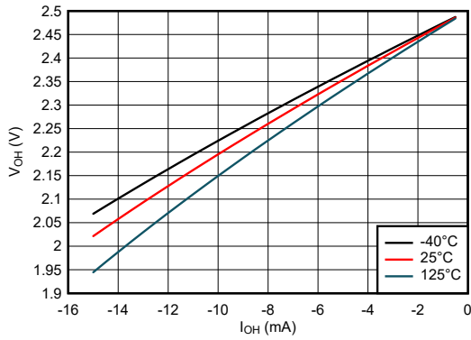
图 5-20. 高电平状态下输出电压与电流间的关系 (2.5V 电源)
