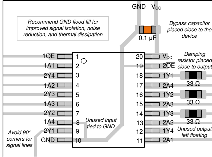
图 10-3. SN74LV8T244 采用 TSSOP 封装的示例布局
