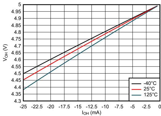
图 5-16. 高电平状态下输出电压与电流间的关系 (5V 电源)
