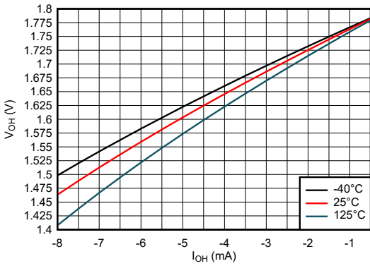
图 5-22. 高电平状态下输出电压与电流间的关系 (1.8V 电源)
