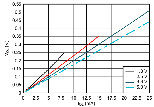
图 5-15. 低电平状态下输出电压与电流间的关系
