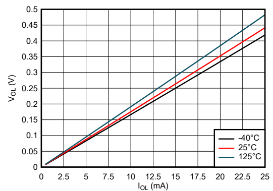
图 5-17. 低电平状态下输出电压与电流间的关系 (5V 电源)
