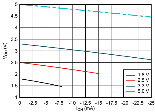
图 5-14. 高电平状态下输出电压与电流间的关系
