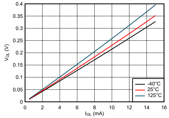
图 5-21. 低电平状态下输出电压与电流间的关系 (2.5V 电源)
