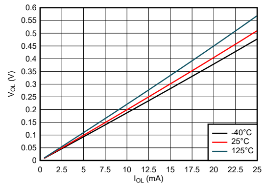
图 5-19. 低电平状态下输出电压与电流间的关系 (3.3V 电源)
