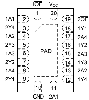
图 4-2. SN74LV8T244 RKS 封装；20 引脚 TSSOP (顶视图)
