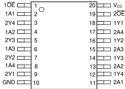
图 4-1. PW 或 DGS 封装，20 引脚 TSSOP 或 VSSOP (顶视图)
