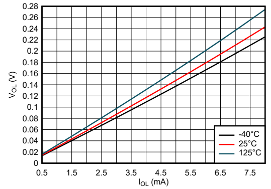
图 5-23. 低电平状态下输出电压与电流间的关系 (1.8V 电源)
