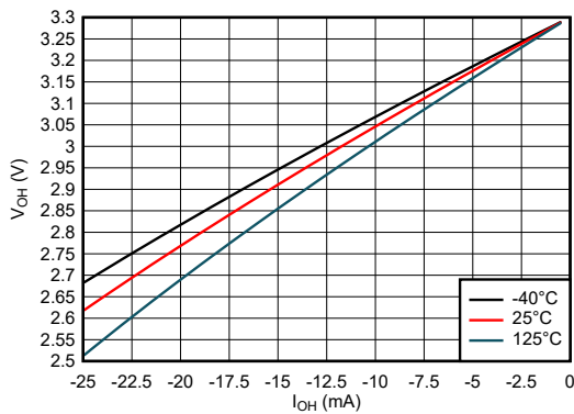
图 5-18. 高电平状态下输出电压与电流间的关系 (3.3V 电源)
