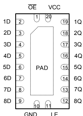
图 4-1. SN74LV8T573-Q1 RKS 封装 (顶视图)
