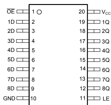
图 4-2. SN74LV8T573-Q1 PW、DGS 封装 (顶视图)
