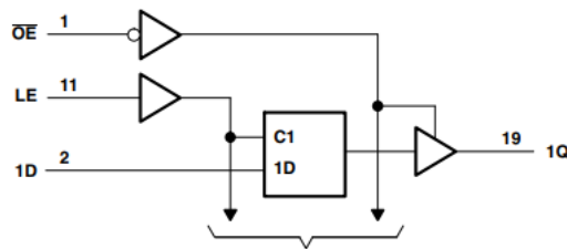
图 7-1. 其他 7 个通道的逻辑图 (正逻辑)
