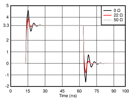
图 8-2. 使用不同阻尼电阻器 ( R_d ) 值的接收器模拟信号完整性
