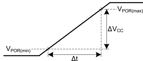
图 7-2. 已知上电状态的电源 (V CC ) 斜坡特性
