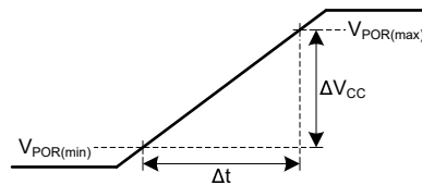
图 7-2. 已知上电状态的电源 (V CC ) 斜坡特性
