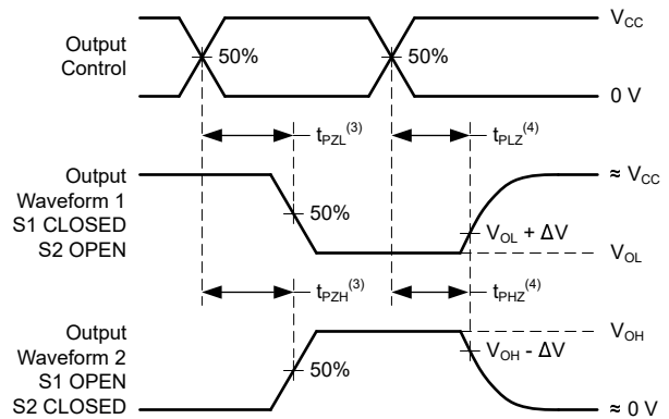
(3) t_{PZL} 和 t_{PZH} 之间的较大者与 t_{en} 相同。
