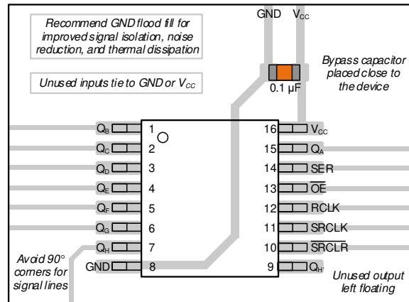
图 8-3. SN74LV8T596 采用 TSSOP 封装的示例布局
