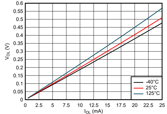
图 5-6. 低电平状态下输出电压与电流间的关系 (3.3V 电源)
