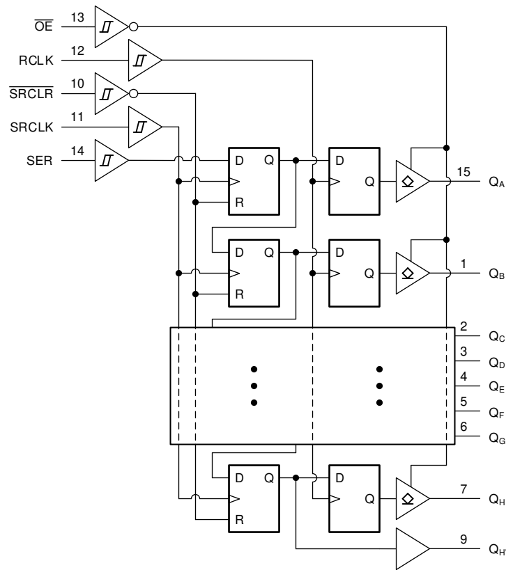
图 7-1. SN74LV8T596 的逻辑图 (正逻辑)
