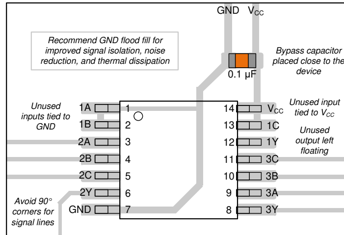
图 8-3. SN74LVC11A-Q1 示例布局
