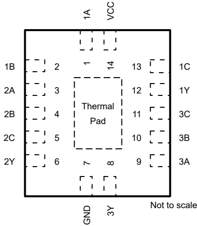
图 4-1. SN74LVC11A-Q1 BQA 封装，14 引脚 WQFN (顶视图)
