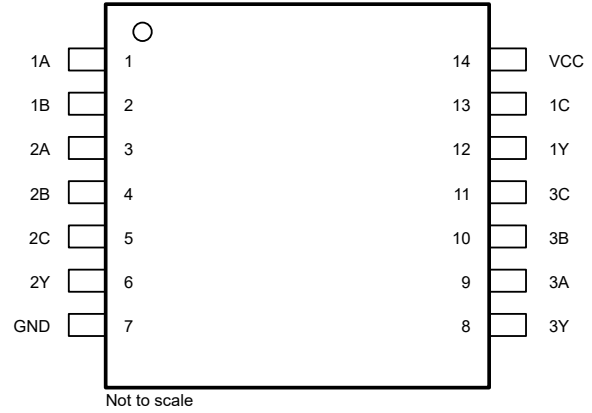
图 4-2. SN74LVC11A-Q1 D 或 PW 封装，14 引脚 SOIC 或 TSSOP (顶视图)
