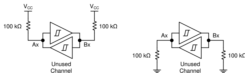
图 7-2. 未使用收发器通道的正确端接
