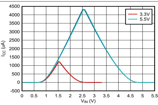
图 5-2. 电源电流与输入电源电压 (3.3V 至 5.5V) 间的关系
