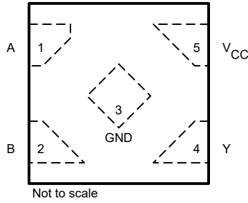
图 4-1. DTX 封装 5 引脚 X2SON (顶视图)
