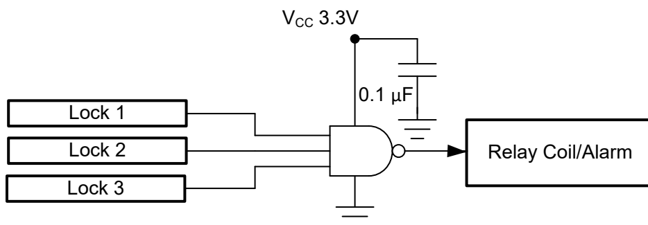
图 8-1. 典型应用图
