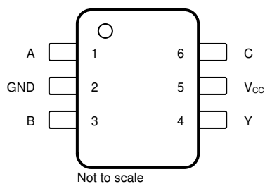
图 4-1. DCK 封装，6 引脚 SC-70（俯视图）
