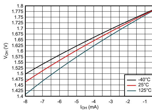
图 5-9. 高电平状态下输出电压与电流间的关系 (1.8V 电源)
