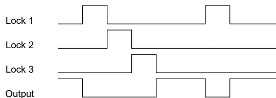
图 8-2. 互锁信号和逻辑输出
