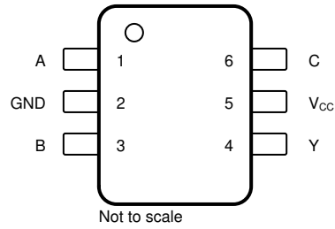
图 4-1. DCK 或 DBV 封装，6 引脚 SC-70 或 SOT-23（俯视图）
