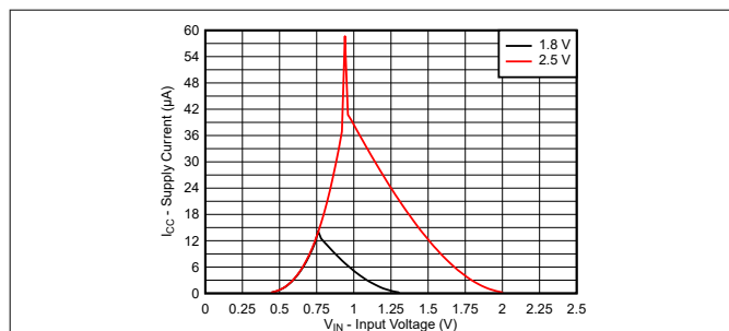
图 5-1. 电源电流与输入电源电压 (1.8V 至 2.5V) 间的关系
