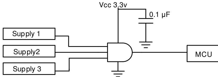
图 8-1. 典型应用图
