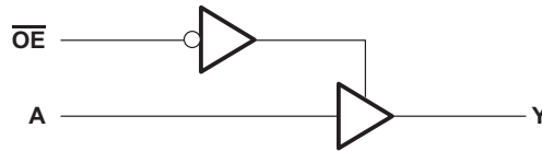
逻辑图
