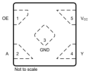
图 4-1. DTX 封装， 5 引脚 X2SON ( 顶视图 )
