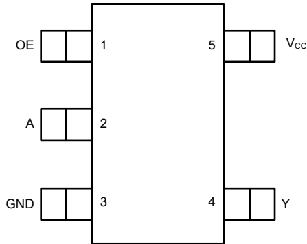
图 4-1. DCK 封装， 5 引脚 SOT-SC70 (顶视图)
